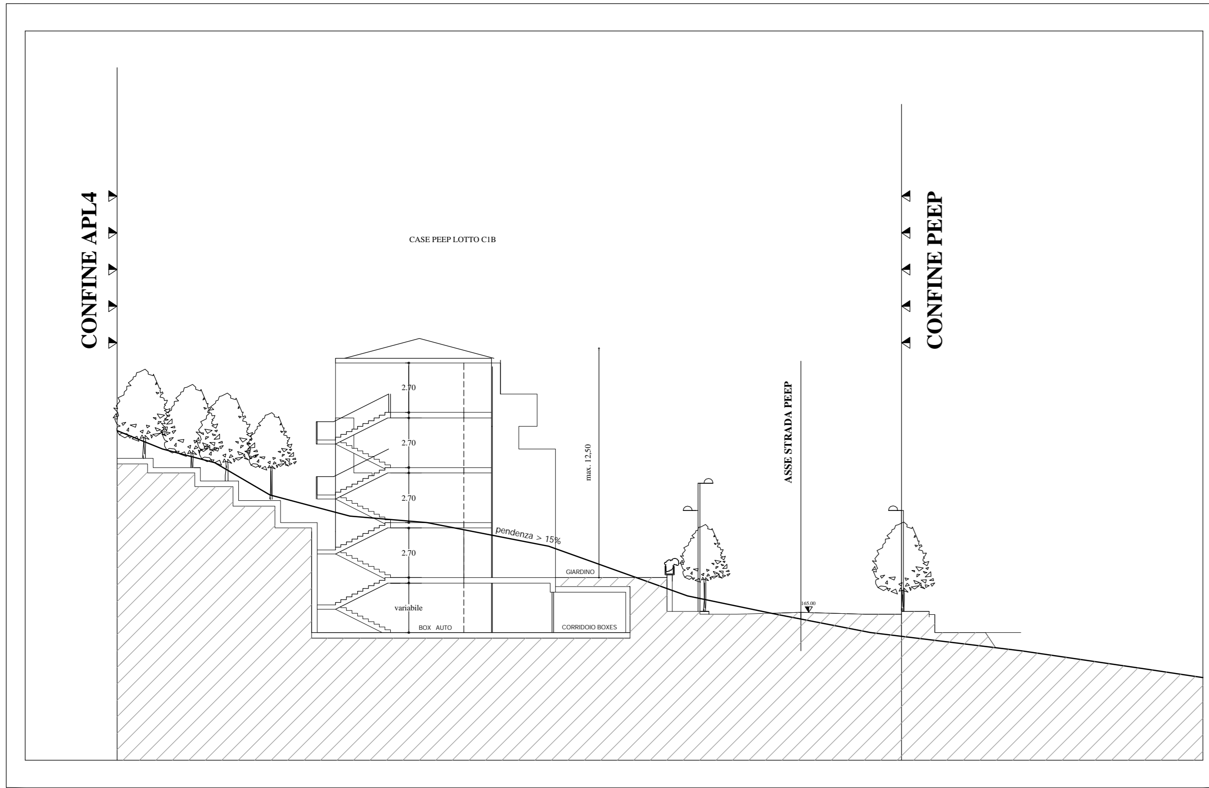
C - C
